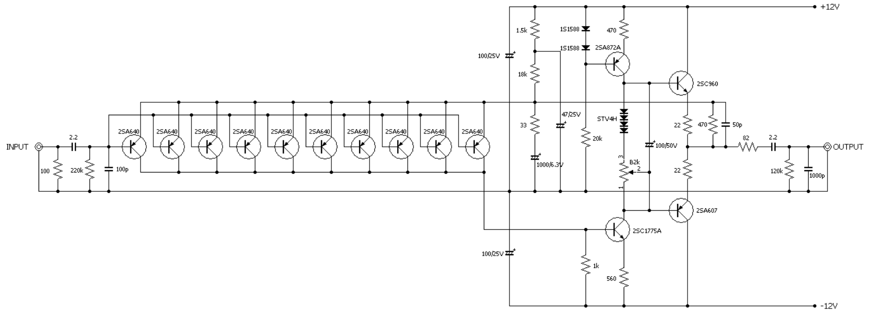
MCヘッドアンプ回路図
