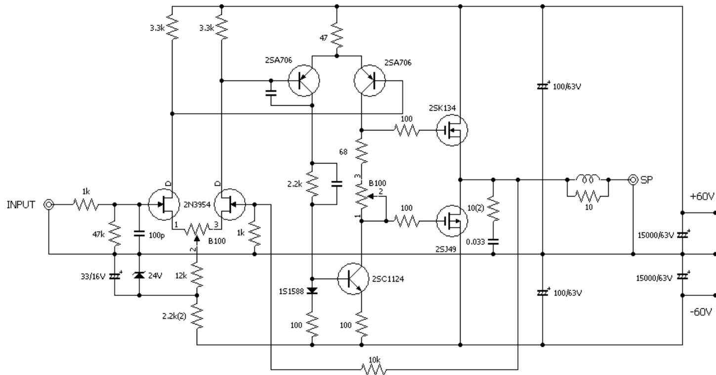
MOS-FETパワーアンプ回路図
