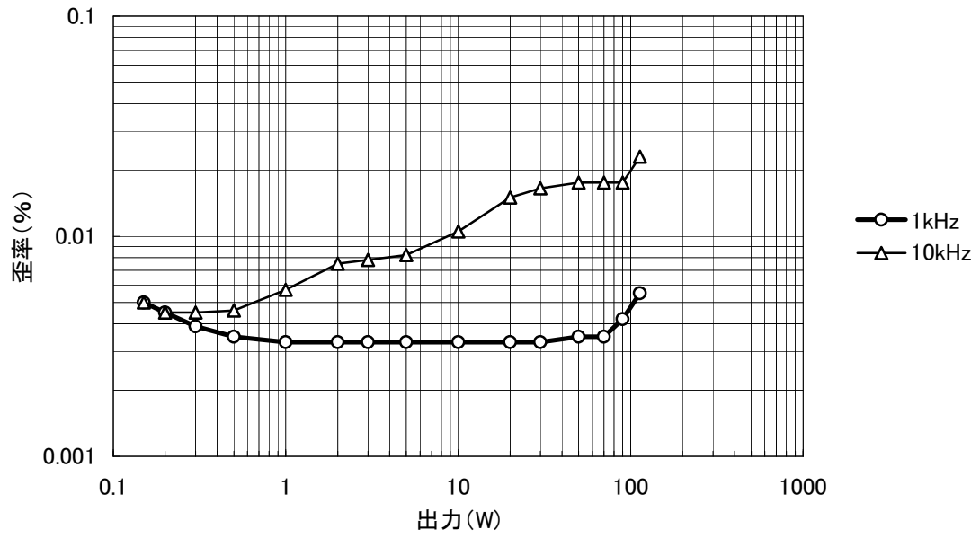
MOS-FETパワーアンプ歪率特性
