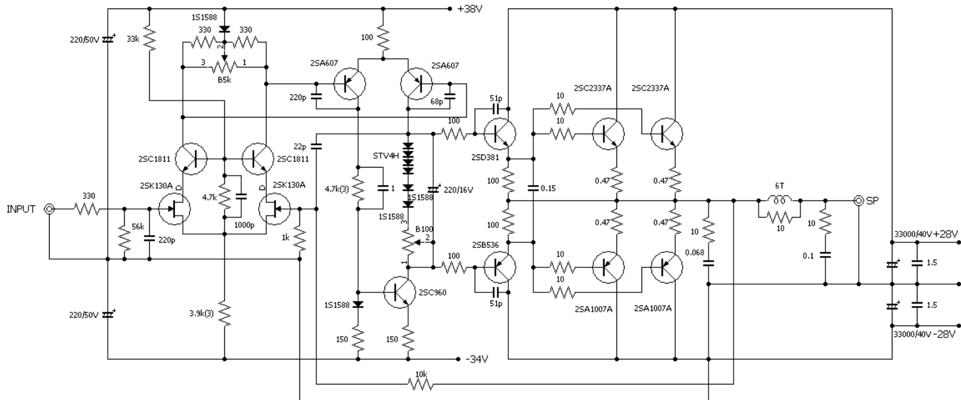
A級30Wパワーアンプ回路図
