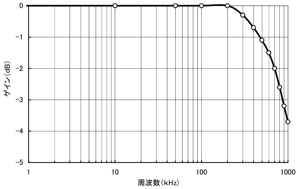
A級30Wパワーアンプ周波数特性
