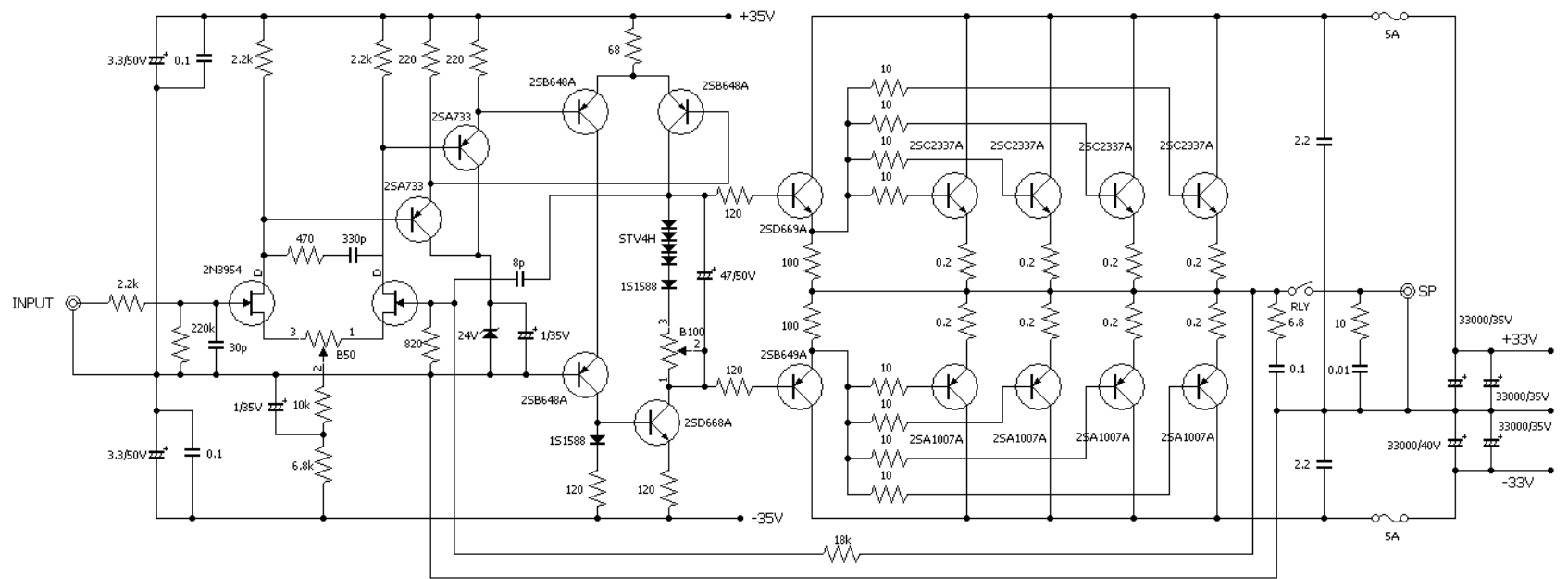
A級50Wパワーアンプ回路図
