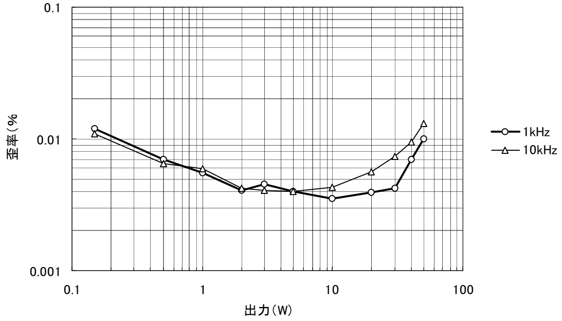
A級50Wパワーアンプ歪率特性
