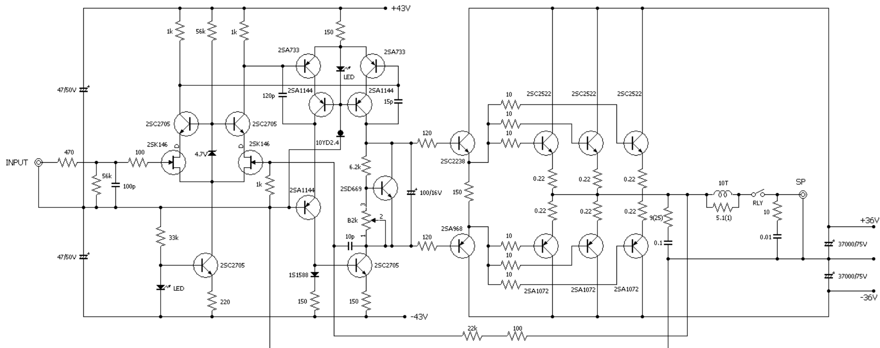
A級60Wパワーアンプ回路図
