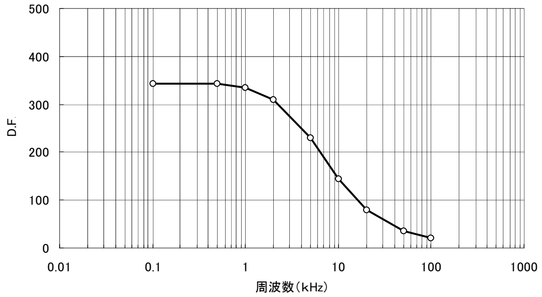
A級60Wパワーアンプダンピングファクター特性
