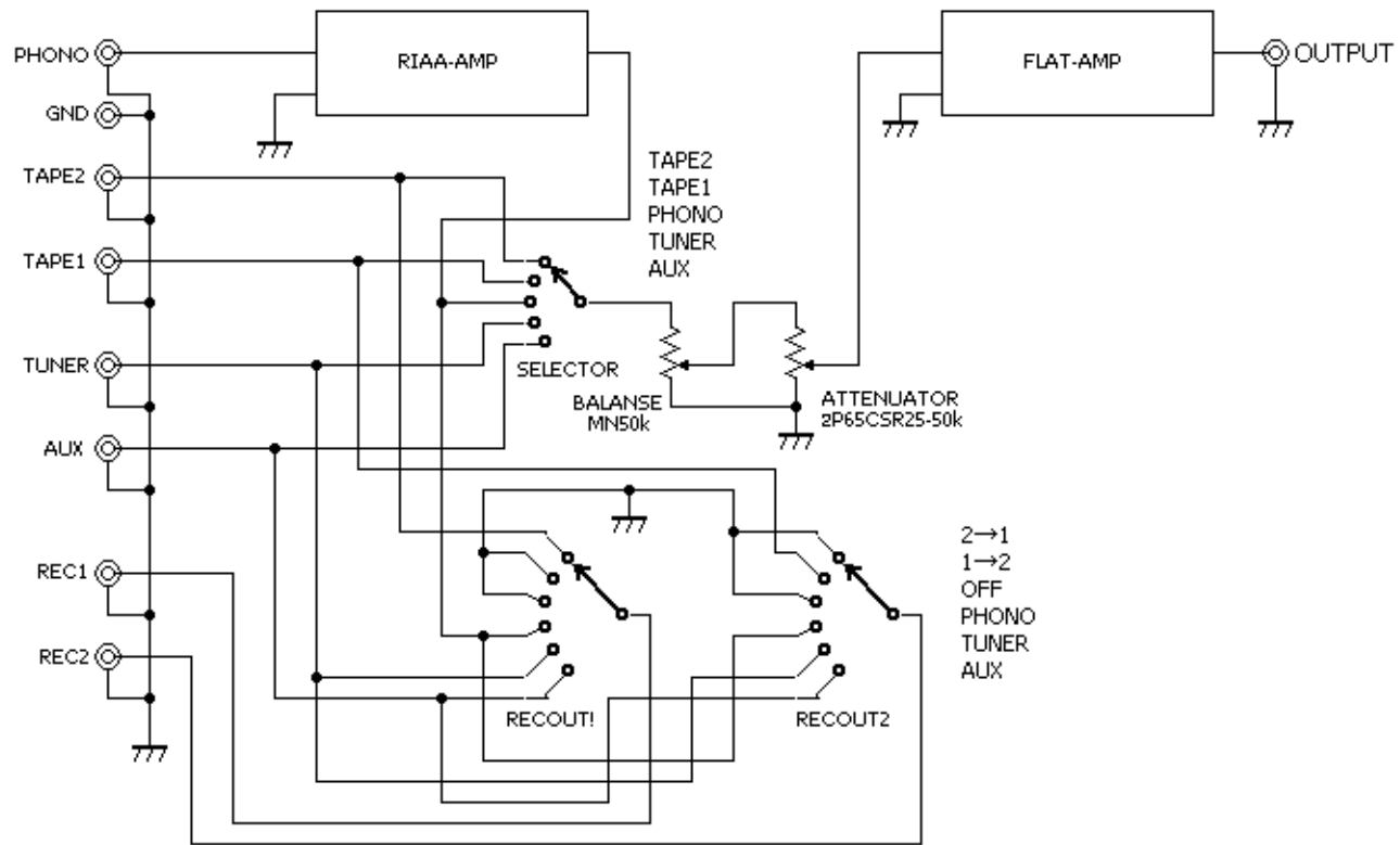
プリアンプ回路図
