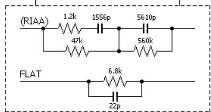
アンプ部回路図
