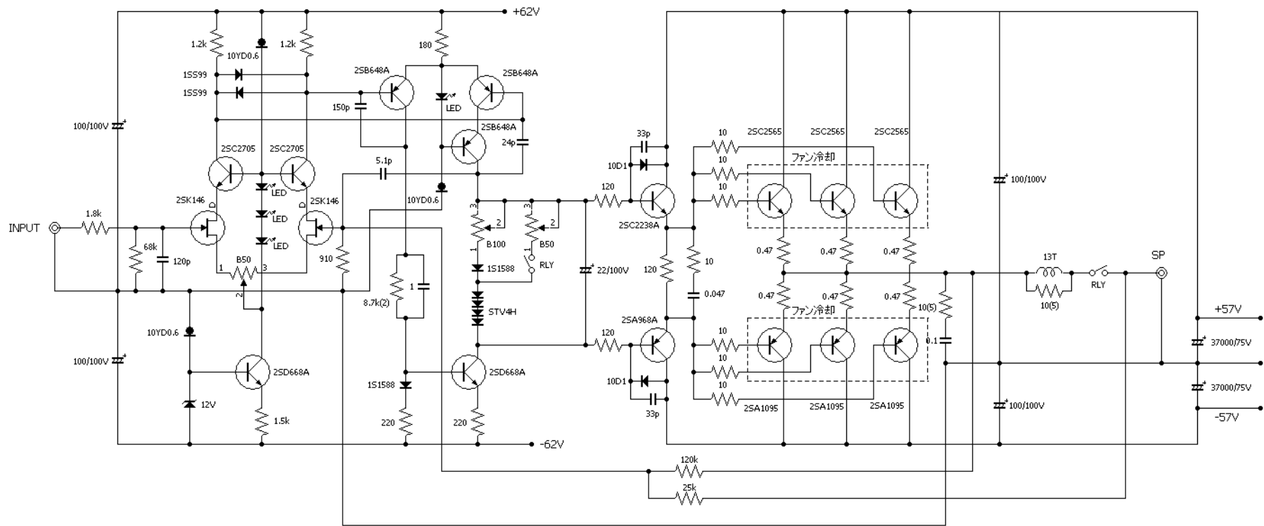
A級100Wパワーアンプ回路図
