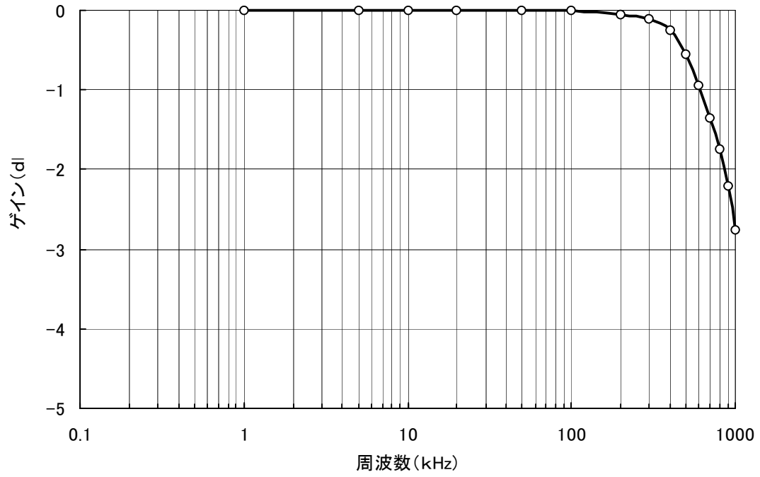
フラットアンプ周波数特性
