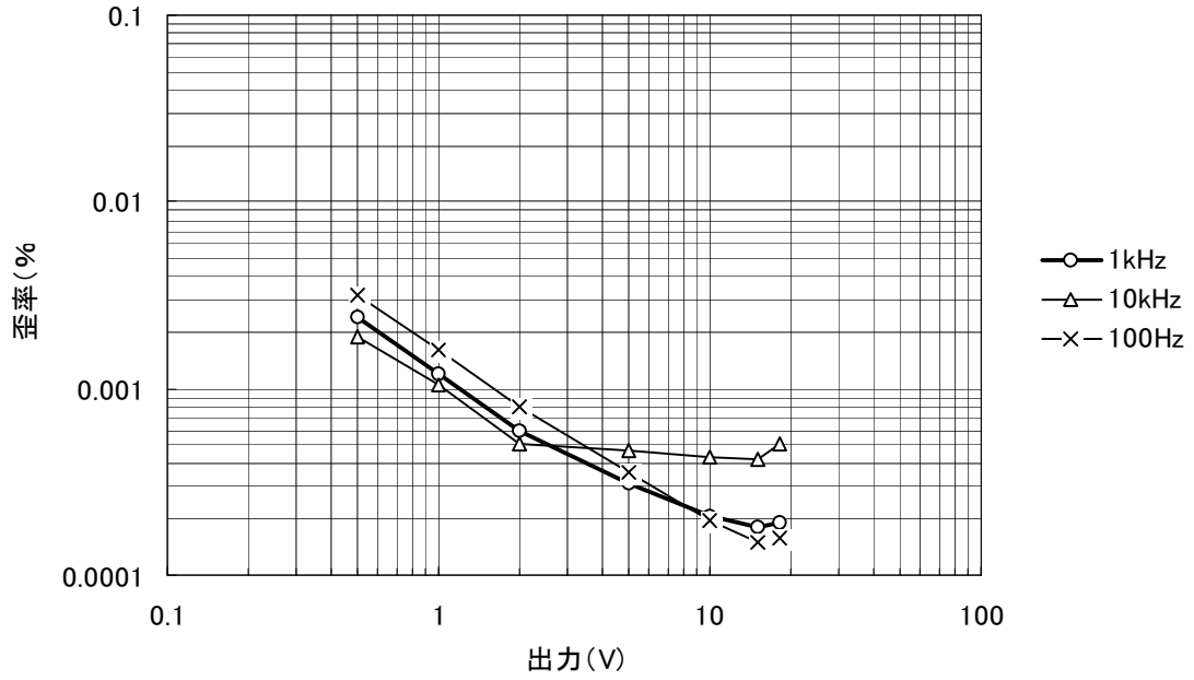
イコライザアンプ歪率特性
