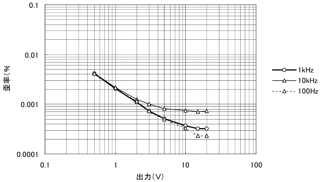
フラットアンプ歪率特性
