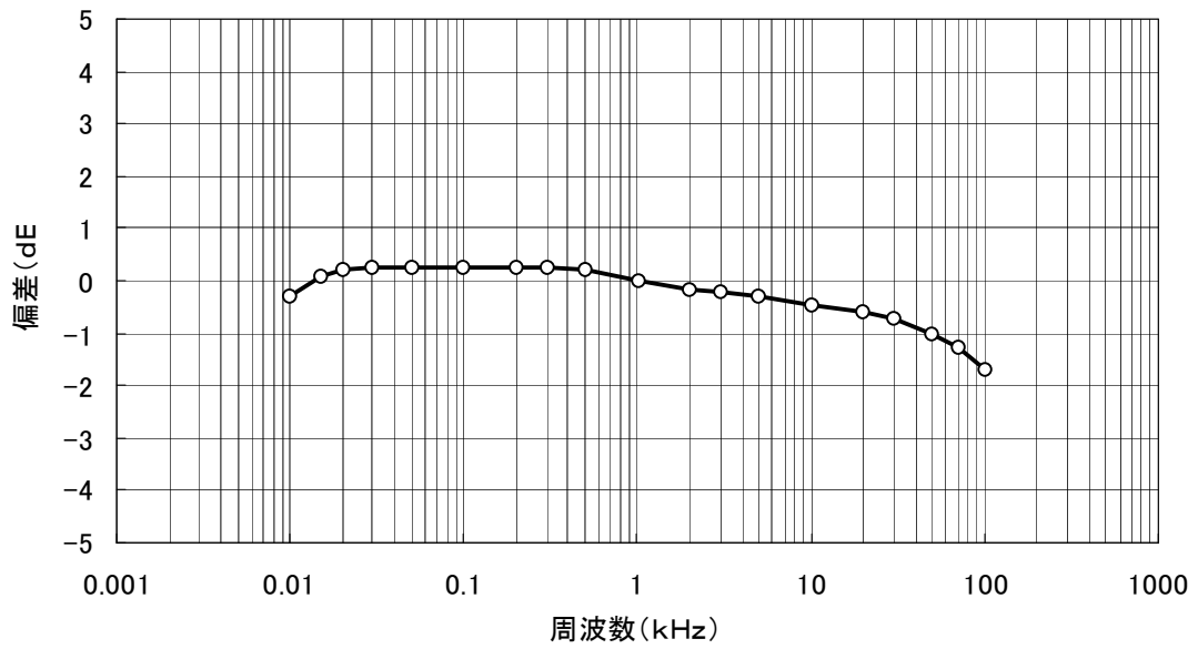
イコライザアンプRIAA偏差
