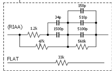
アンプ部回路図
