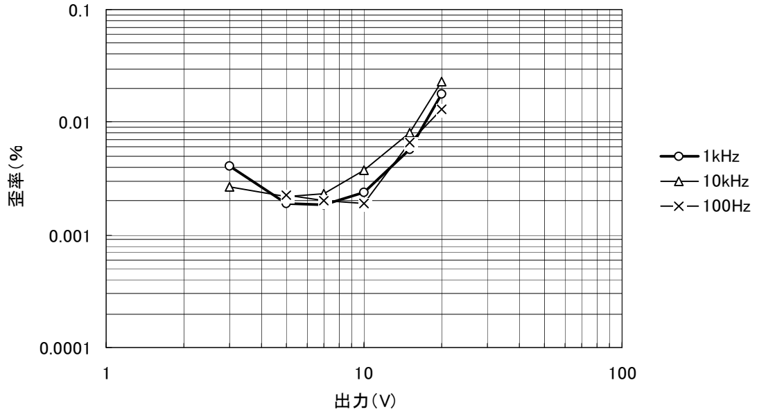
イコライザンプ歪率特性
