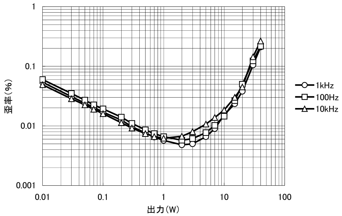
歪率特性
