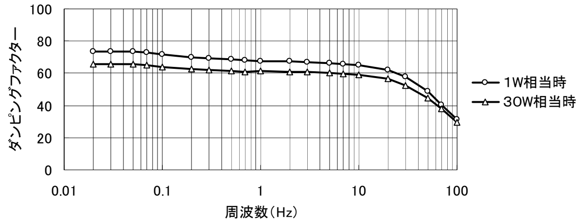
(a) 周波数による変化
