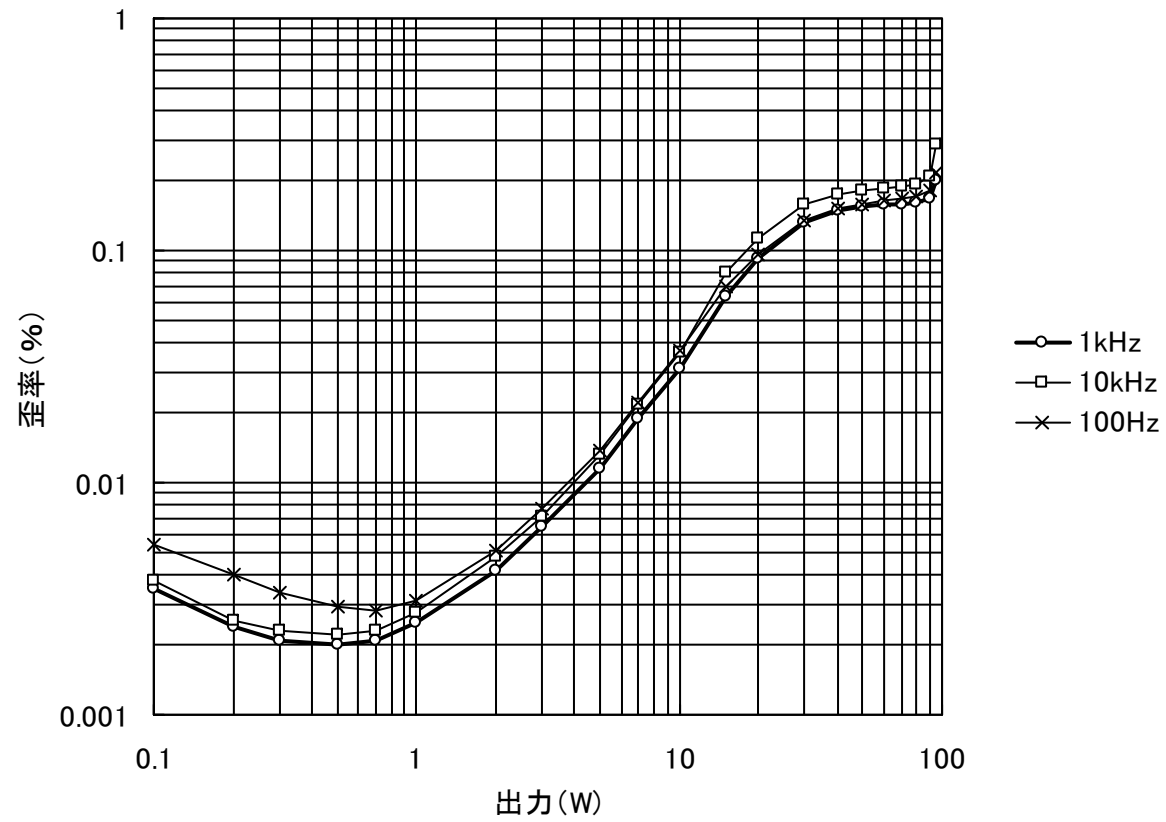
歪率特性(本機単体、負荷8Ω)
