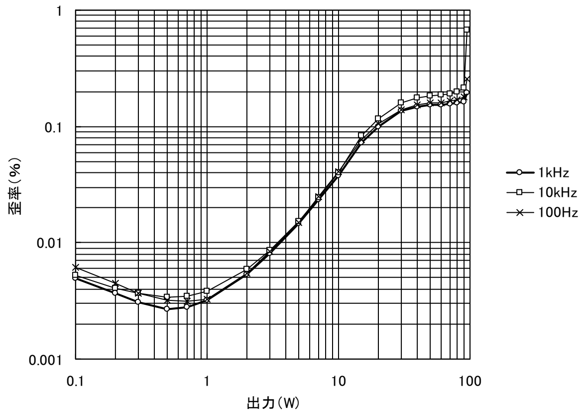
歪率特性(参考、プリアンプ接続、負荷8Ω)
