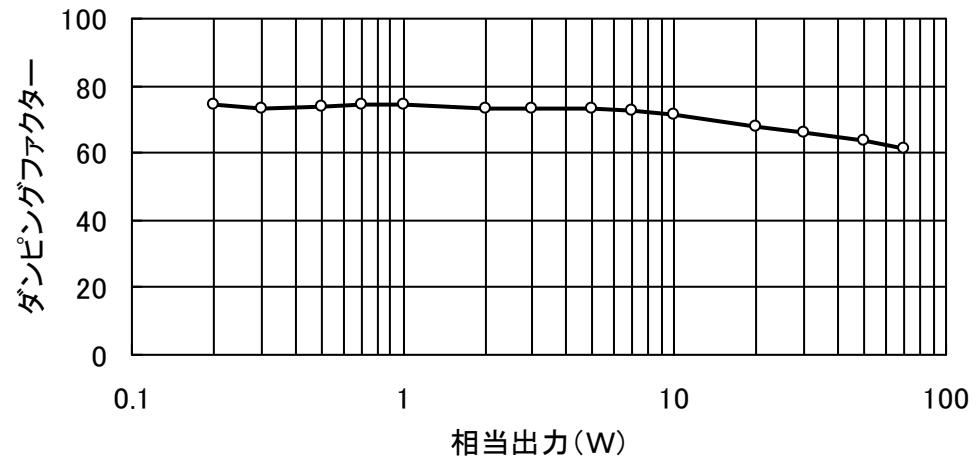
(b) 出力による変化(20Hz)
