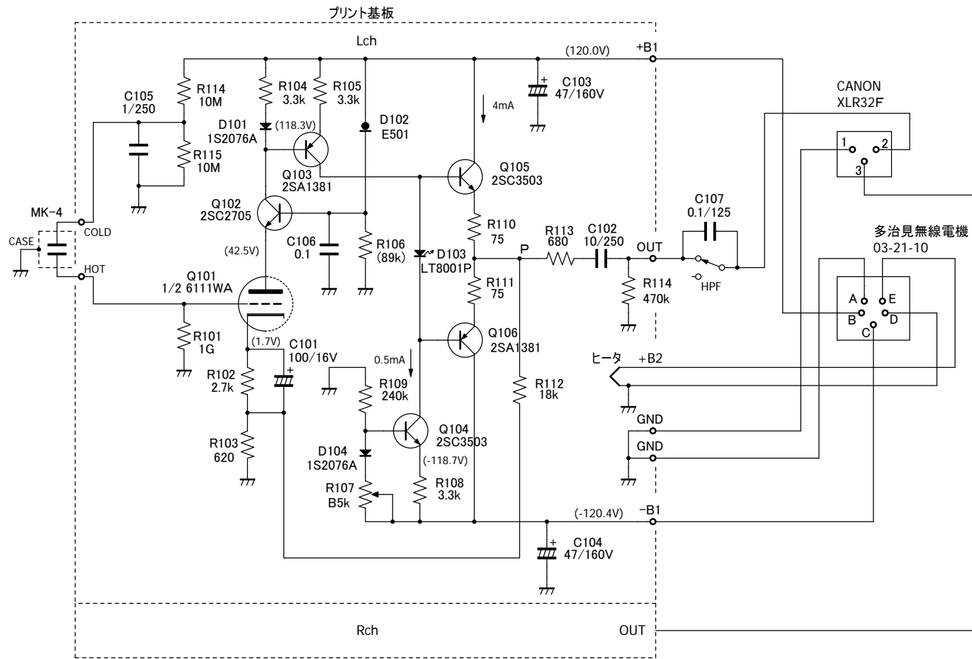
マイクアンプ回路
