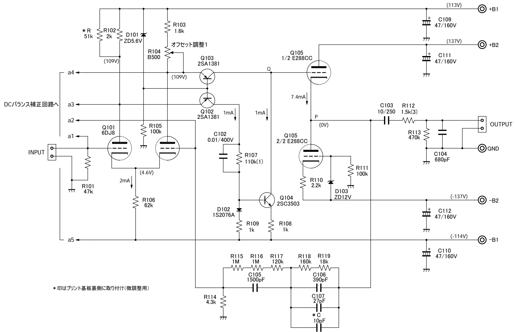
イコライザーアンプ回路
