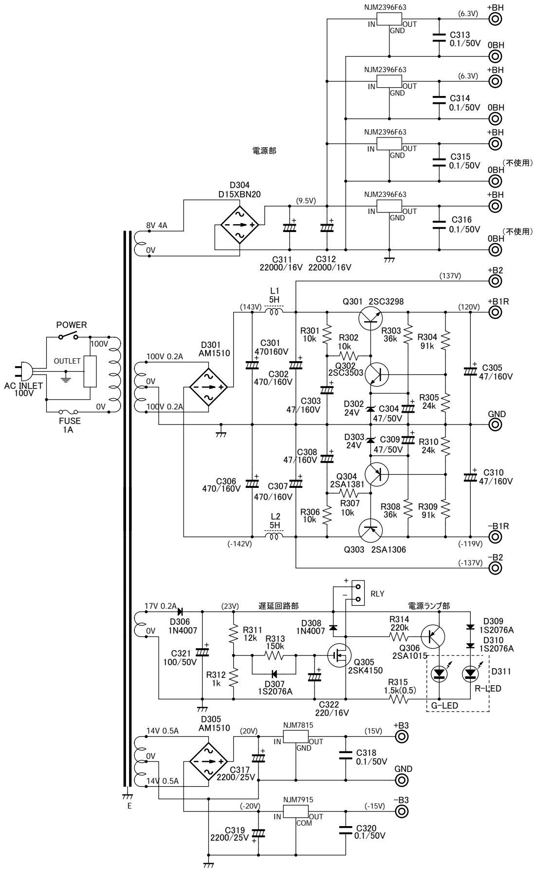
電源部回路
