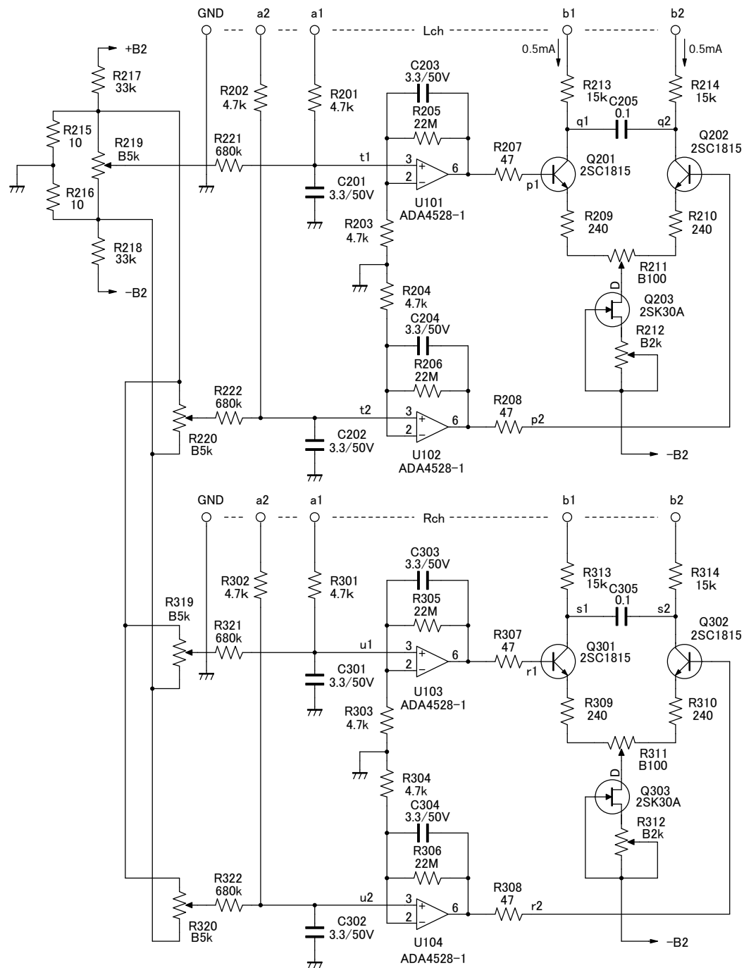
DCバランス補正回路
