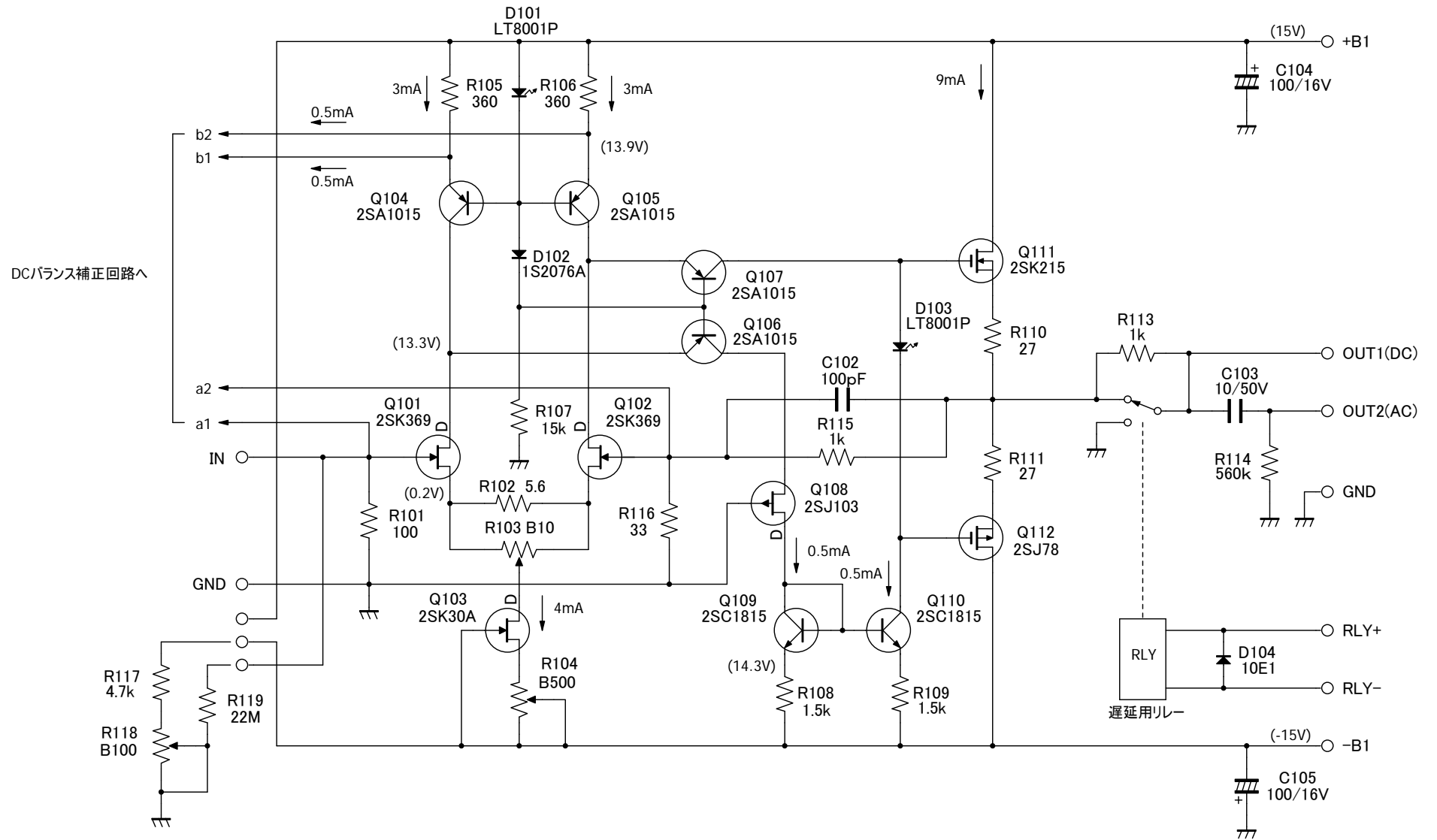
アンプ部回路
