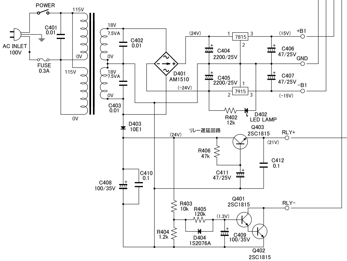
全体回路
