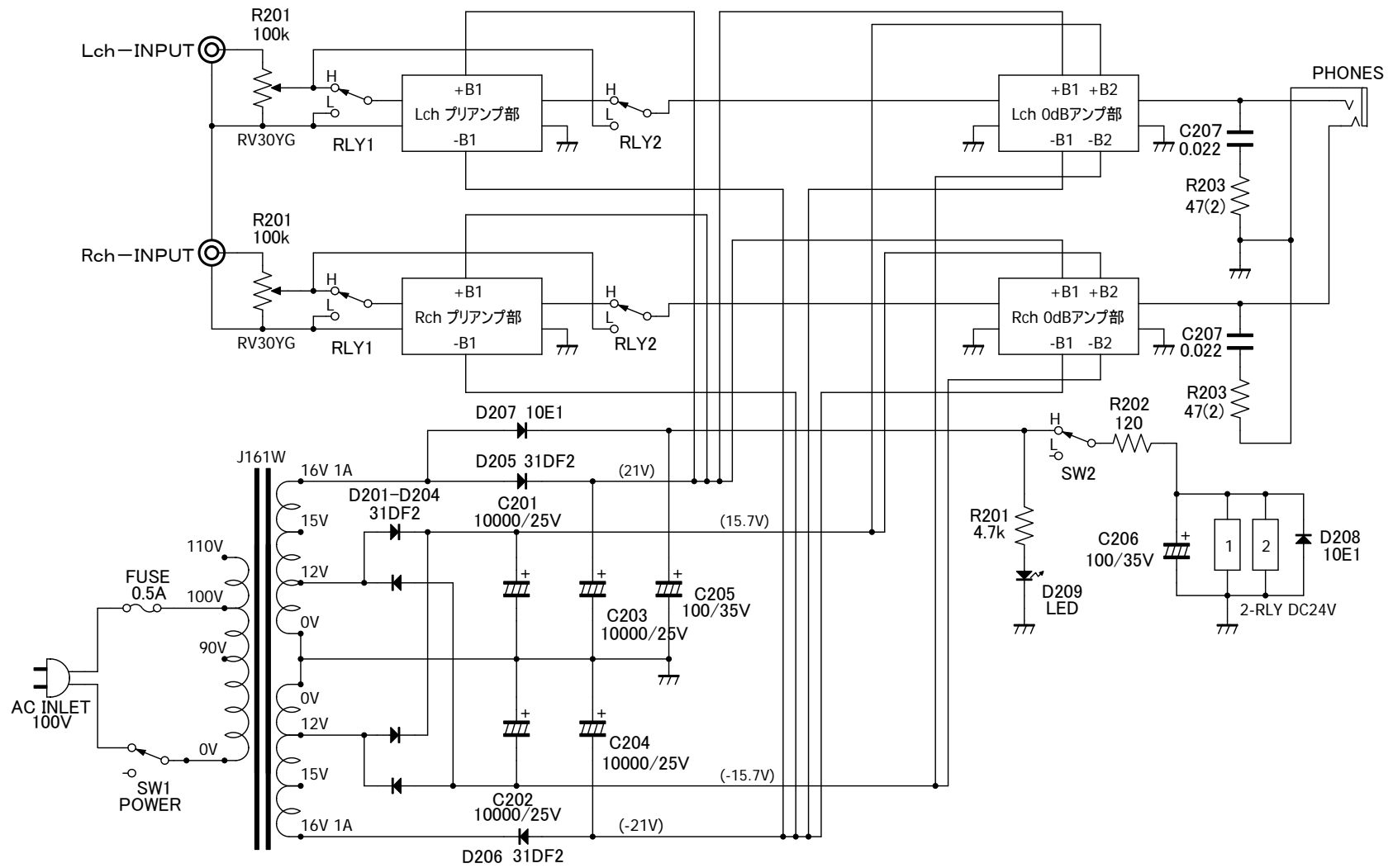
全体回路
