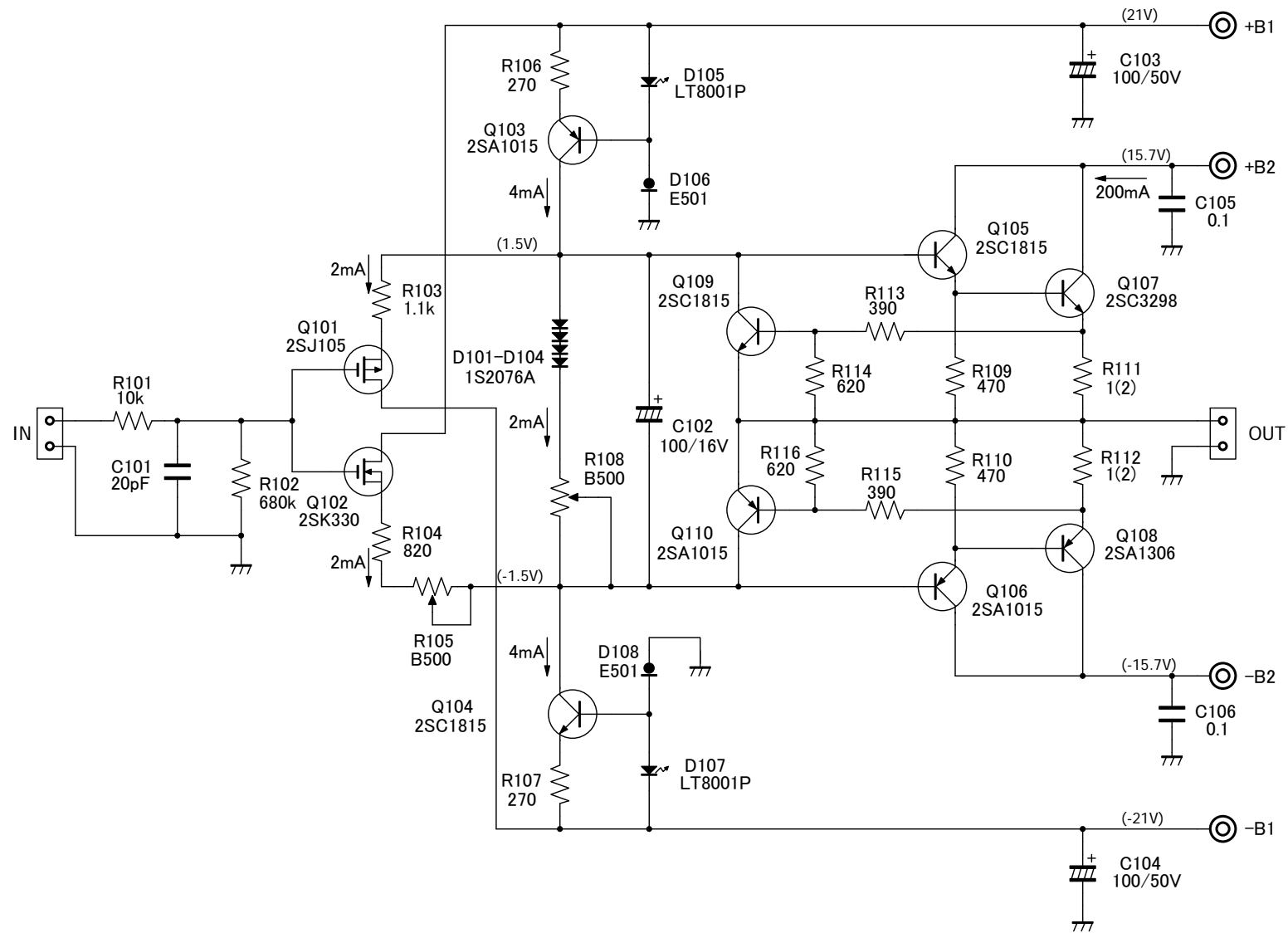
OdBアンプ部回路
