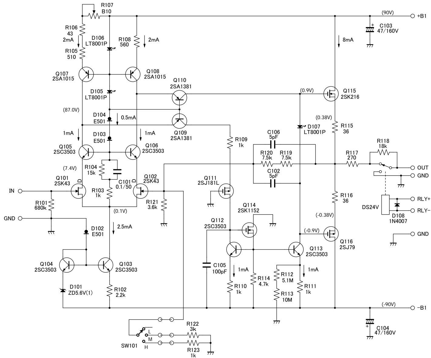
フラットアンプ回路
