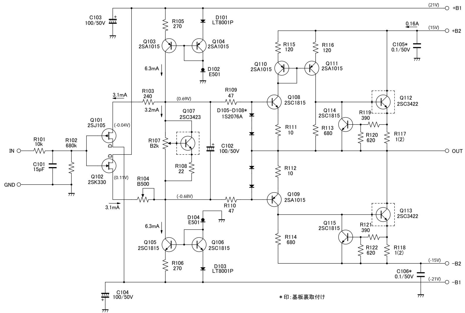
アンプ部回路
