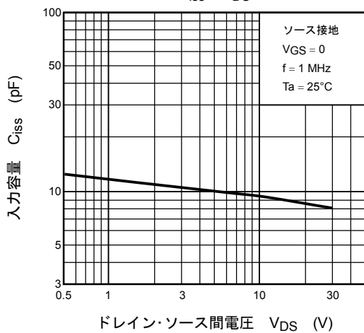
C_{iss} - V_{DS}
