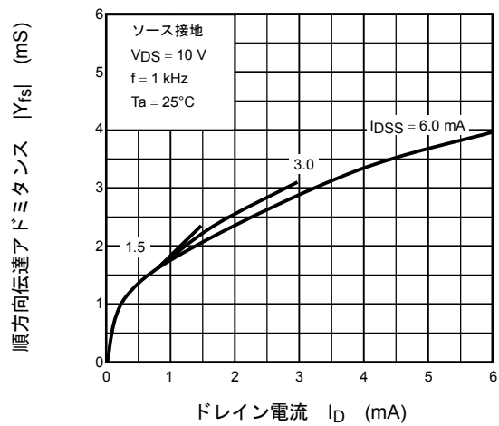
|Y_{fs}| - I_D
