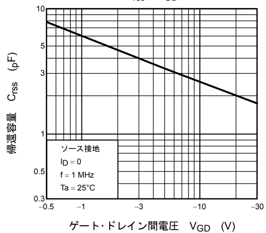
C_{rss} - V_{GD}
