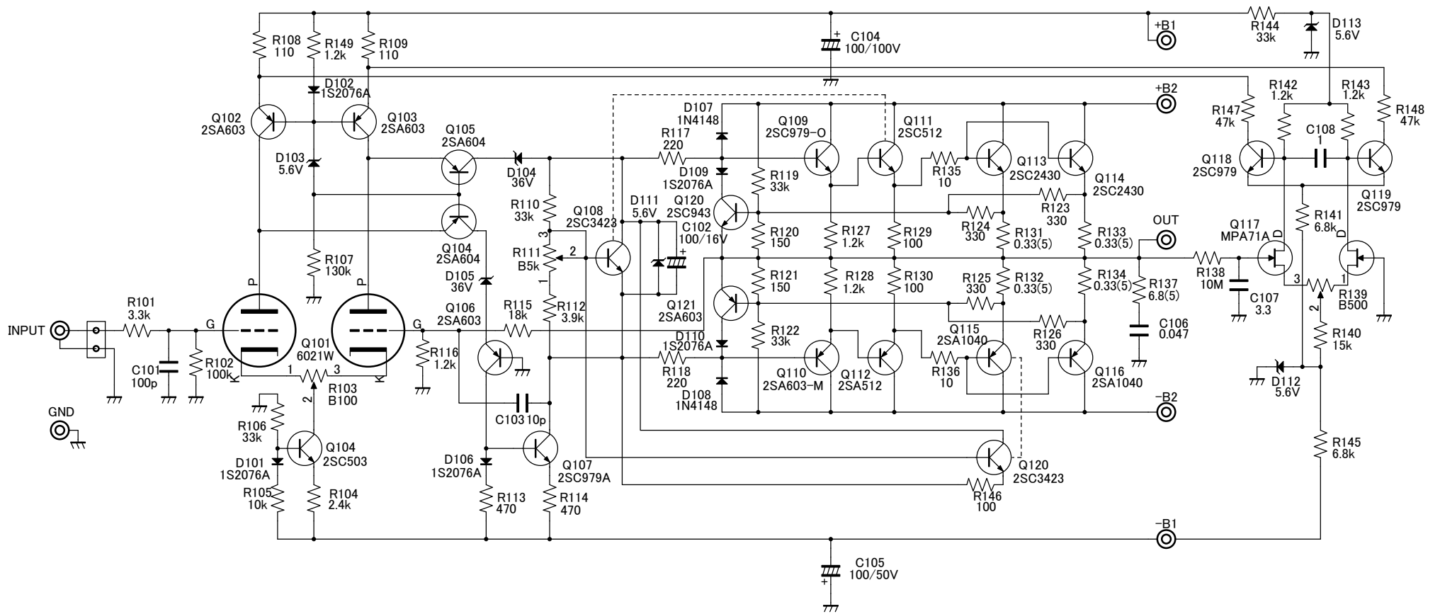
AMP-1301A パワーアンプ回路例
