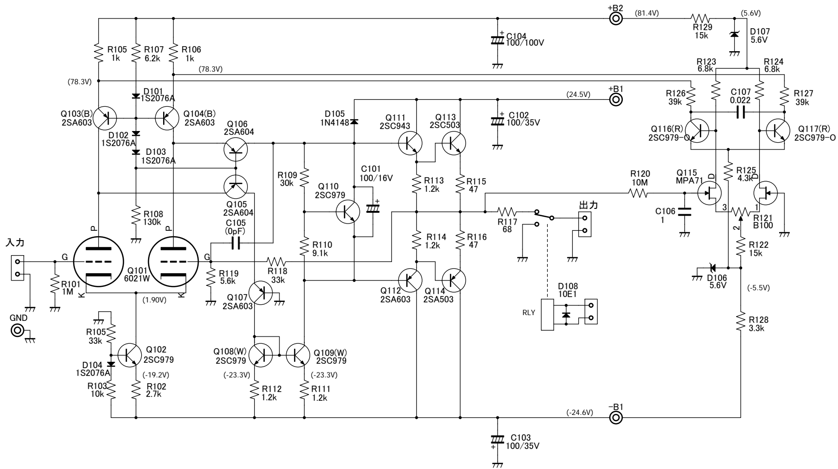
AMP-1401A フラットアンプ回路例
