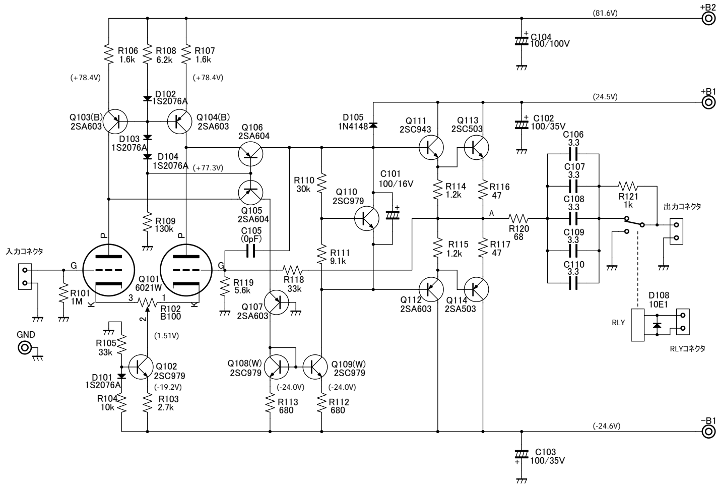
AMP-1401B フラットアンプ回路例
