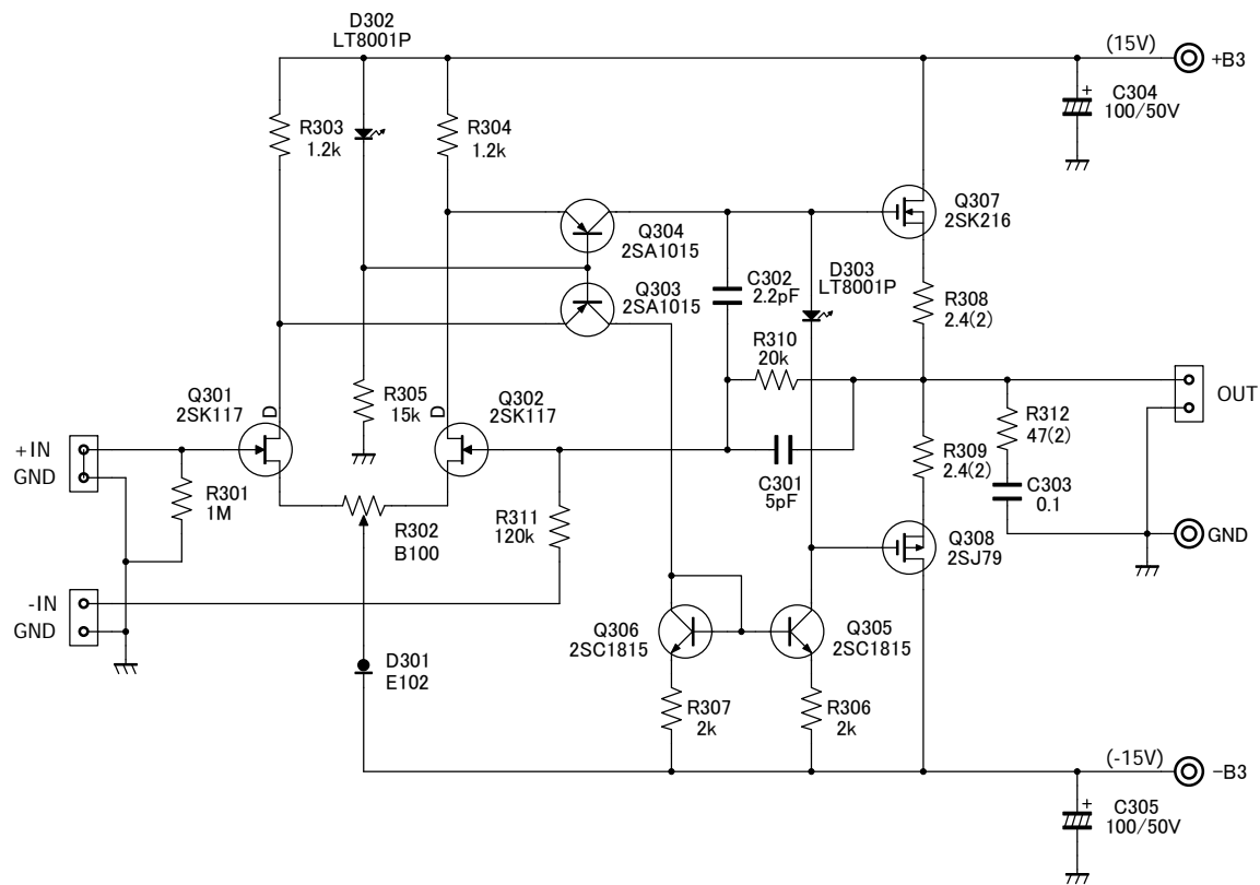
HP-1505A ヘッドホンアンプ回路例
