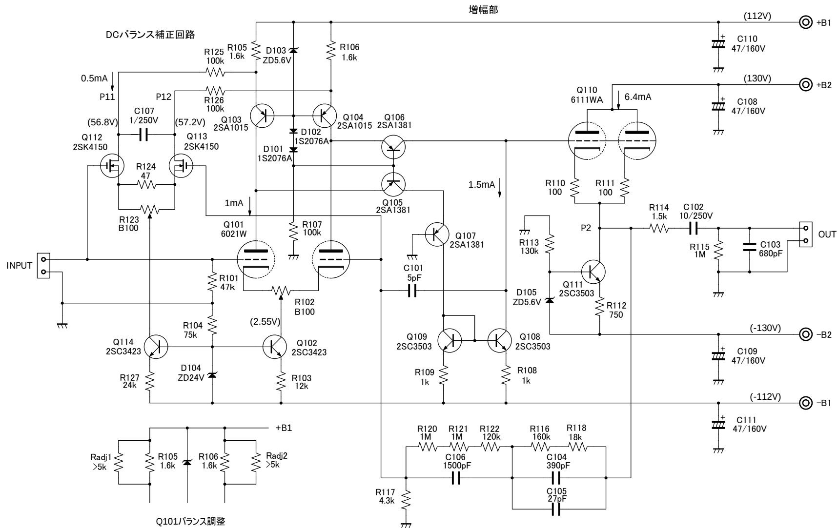
イコライザーアンプ回路
