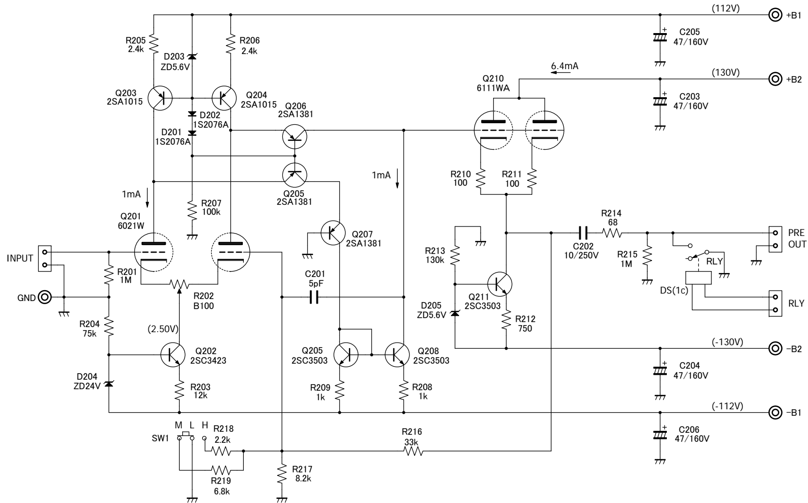
フラットアンプ回路
