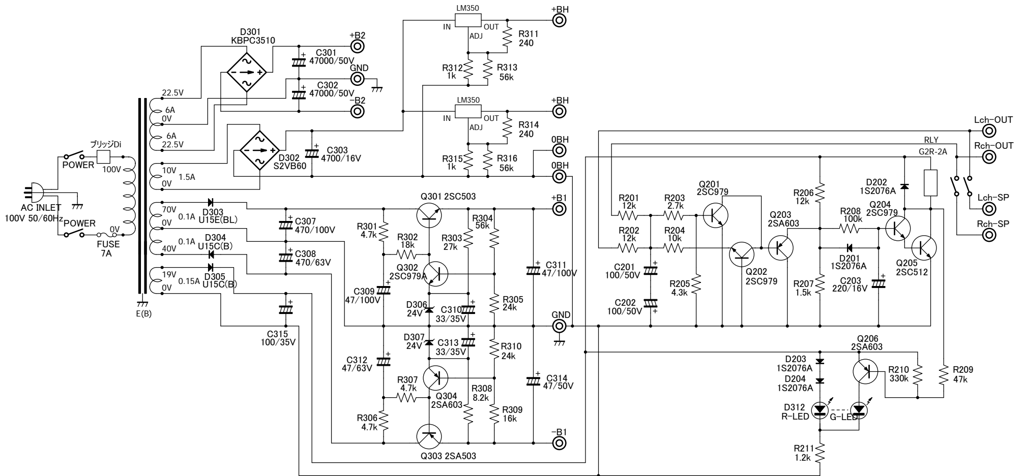
PS-1301A 電源回路例
