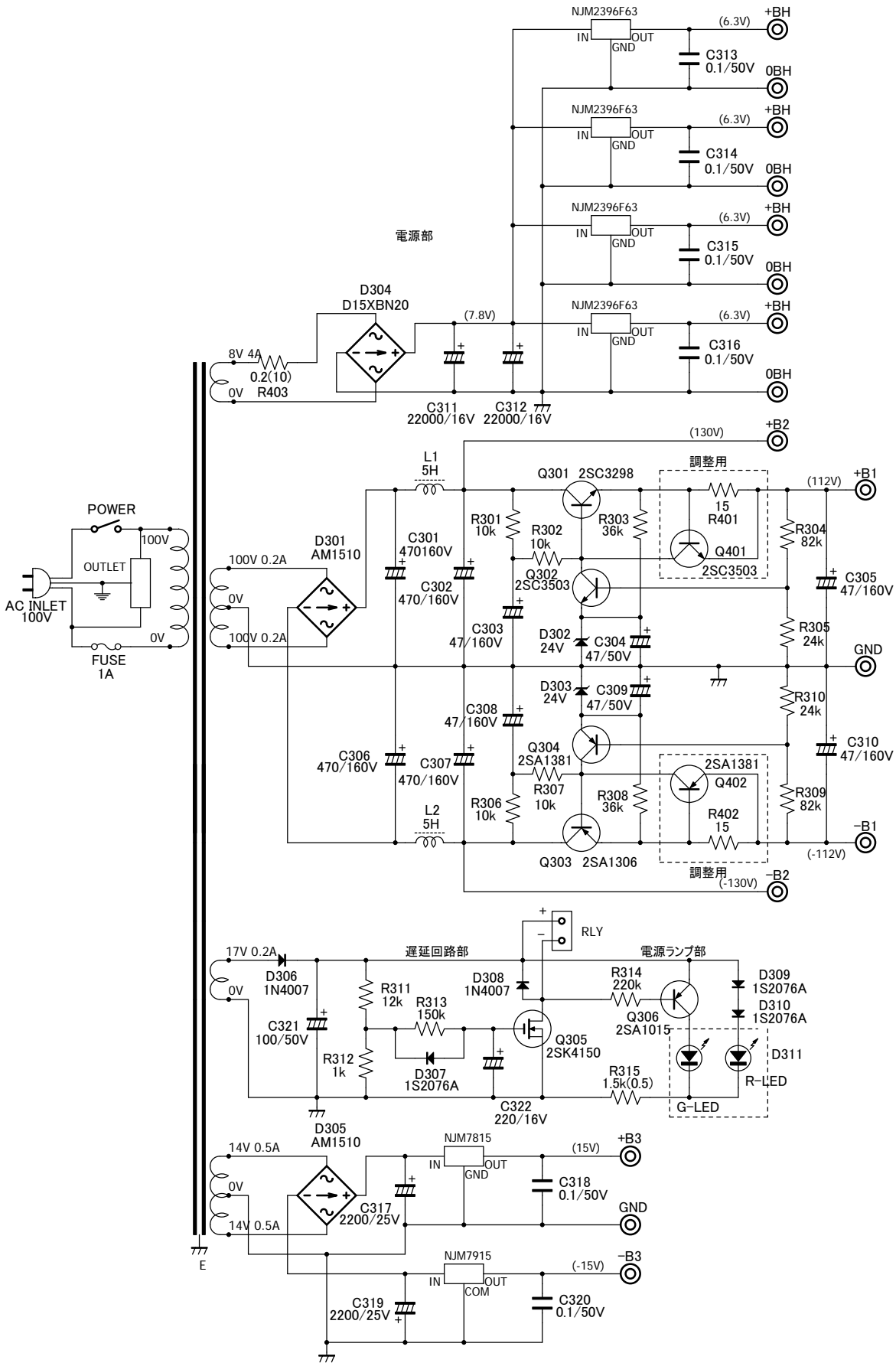
PS-1505A 電源部回路例
